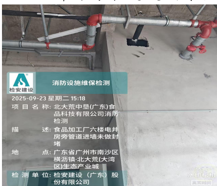
166. 电井房旁管道进墙未做防火封堵。
