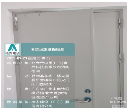
138. 厕所旁楼梯口防火门闭门器缺失。
